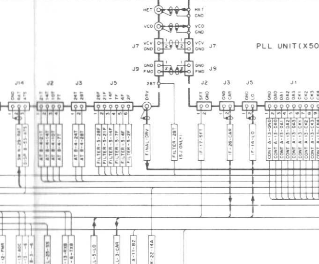
PLL UNIT (X50-2050-00)
