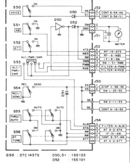
DISPLAY UNIT (X54-1870-00) (B/4)
