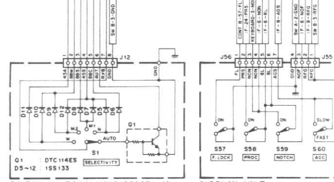
DISPLAY UNIT (X54-1870-00) (D/4)
